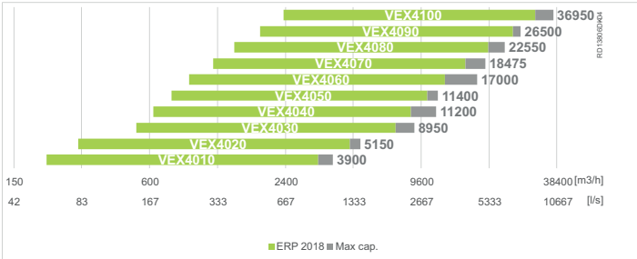
Kapacitetsdiagram
